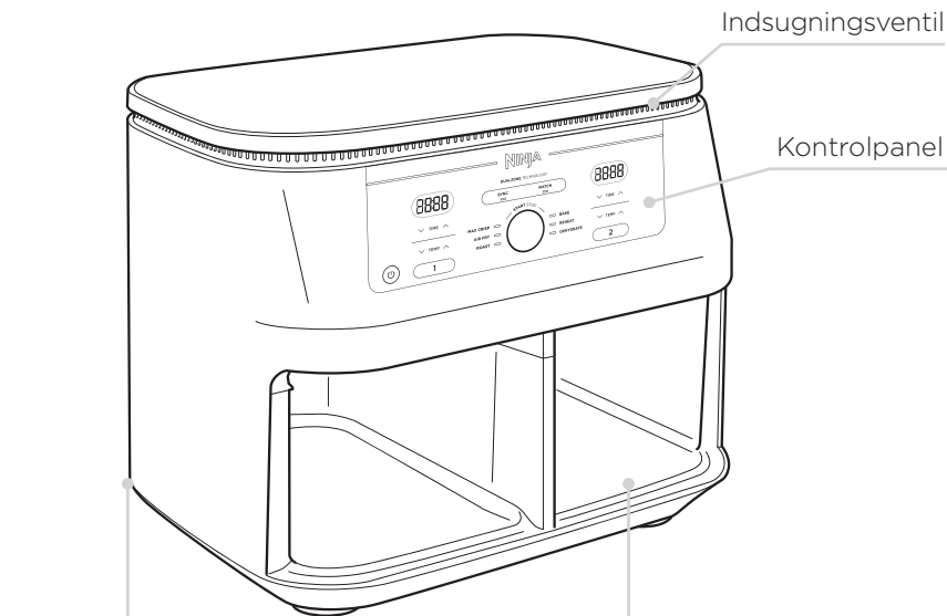
Udluftningsenhed (placeret bagpå)
