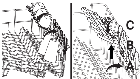
Abbildung 8: Höhenverstellbare Ablage am oberen Korb
